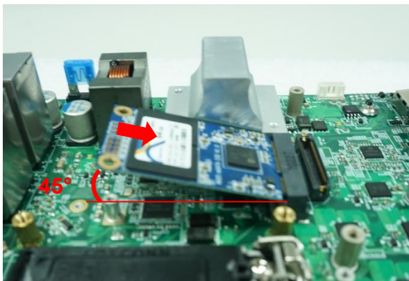
CN3,4,5,6 slot
